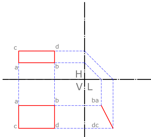
PLANO VERTICAL PERFIL
