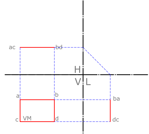
PLANO VERTICAL PARALELO
