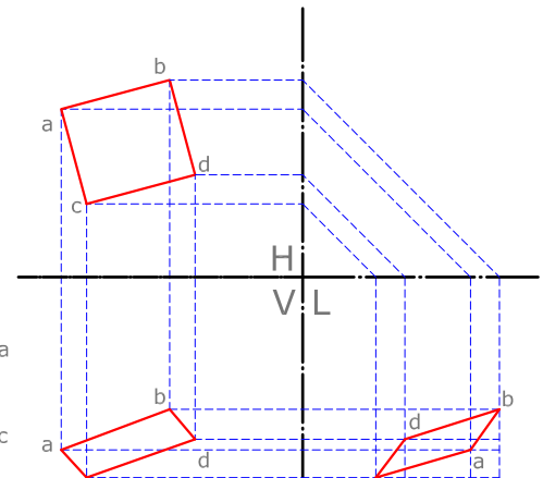
PLANO VERTICAL INCLINADO PERFIL
