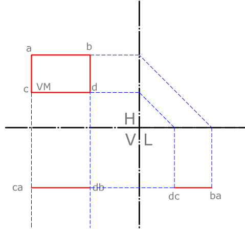
PLANO HORIZONTAL PERFIL
