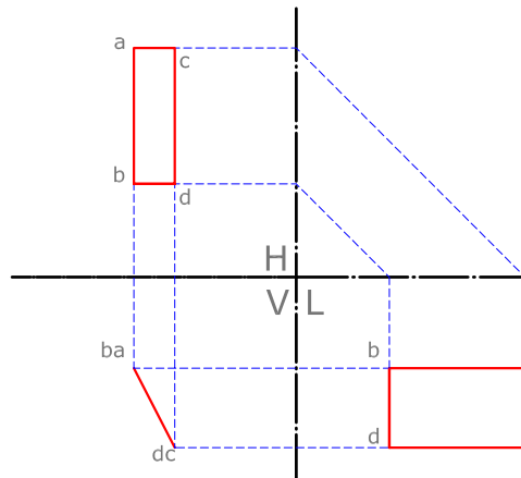
PLANO VERTICAL INCLINADO
