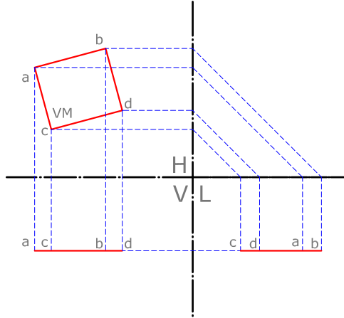
PLANO HORIZONTAL INCLINADO
