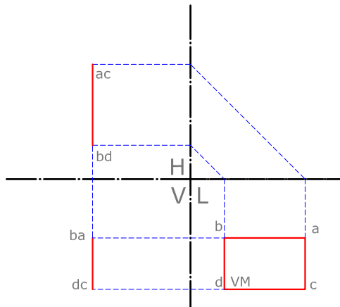
PLANO HORIZONTAL INCLINADO
